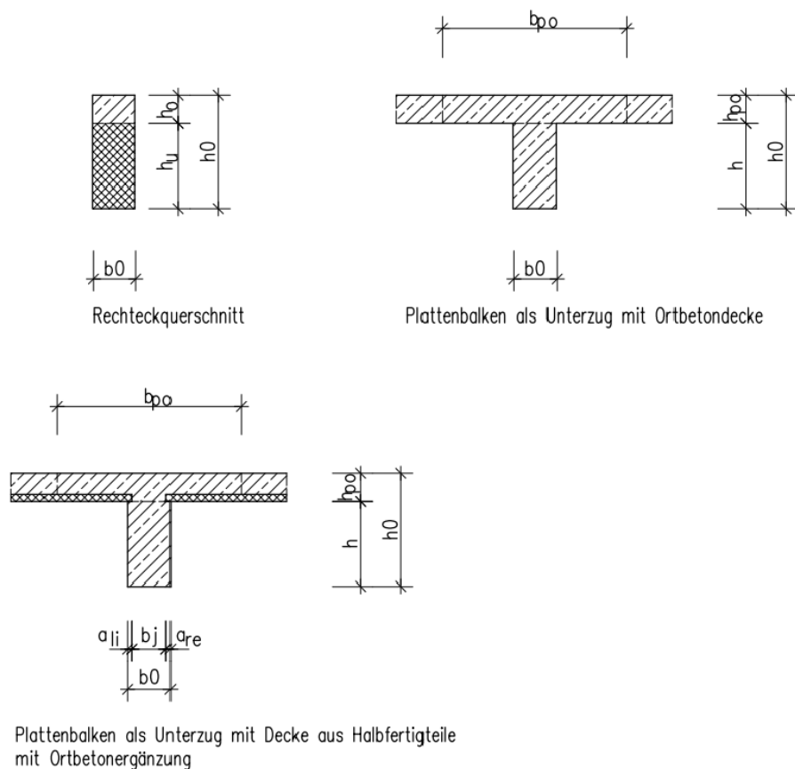
Bild 1: mögliche Systeme
