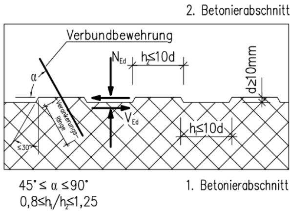
Bild 2: verzahnte Fugenausbildung mit geneigter Verbundbewehrung gem Bild 6.9 aus /1/, /2/
