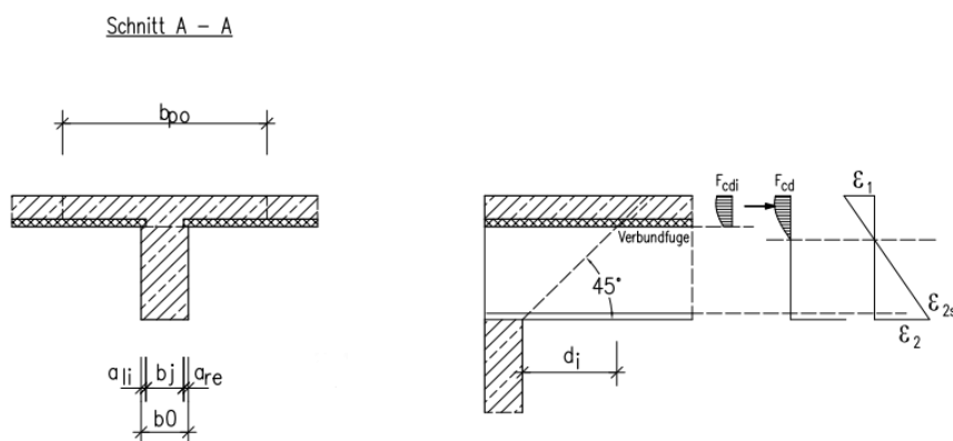
Bild 3: Unterzug mit Darstellung der Schubfuge und Spannungen.
